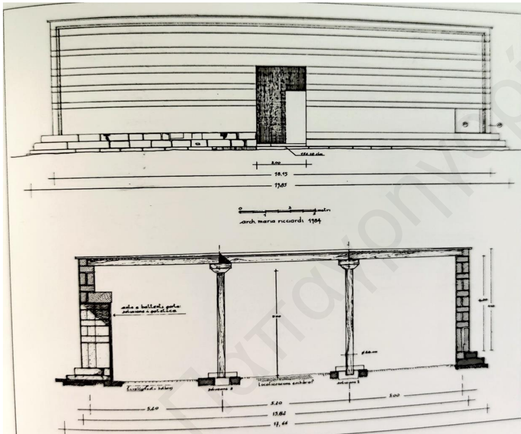
Πύθιον, Αρχαϊκή φάση: όψη και τομή Α-Δ σε ανασύνθεση. Αρχιτ. Μ. Ricciardi. Από Di Vita, Η Γόρτυνα της Κρήτης , 129.
