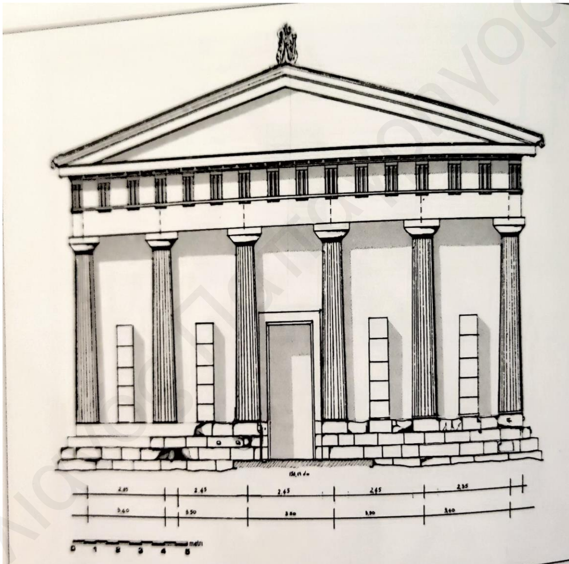
Πύθιον. Η ελληνιστική πρόσοψη, ανασύνθεση της M.Ricciardi. . Από DiVita, Η Γόρτυνα της Κρήτης , 130.
